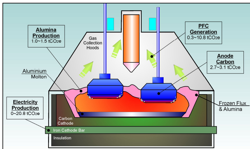
Figura 1: Pontos de emissões de gases em uma célula PFPB. Fonte: Adaptado de IAI (2006).
